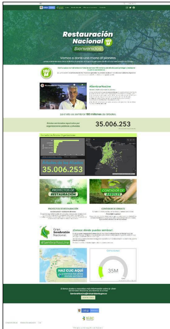
imagen 16 Ejemplo HUB
