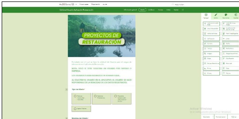
imagen 12 Ejemplo SURVEY123
